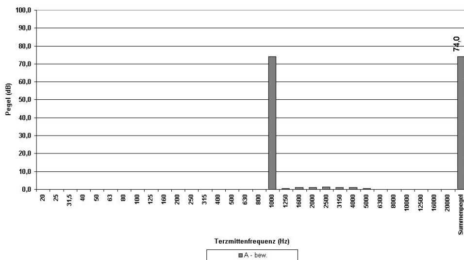
Bild 4a: Schalldruckpegel von schmalbandigem Terzrauschen, Mittenfrequenz 1.000 Hz
